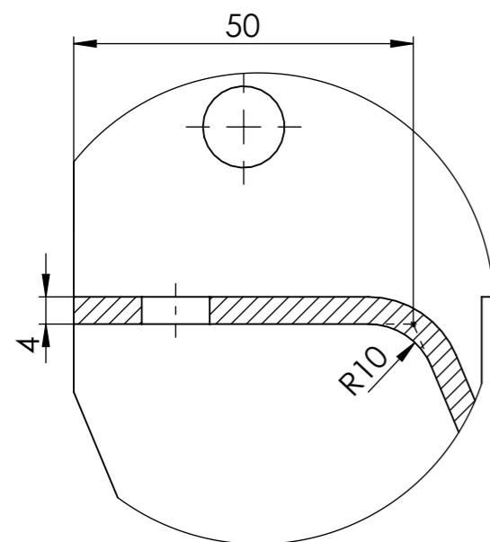
Detalj C Razmera 1 : 1
