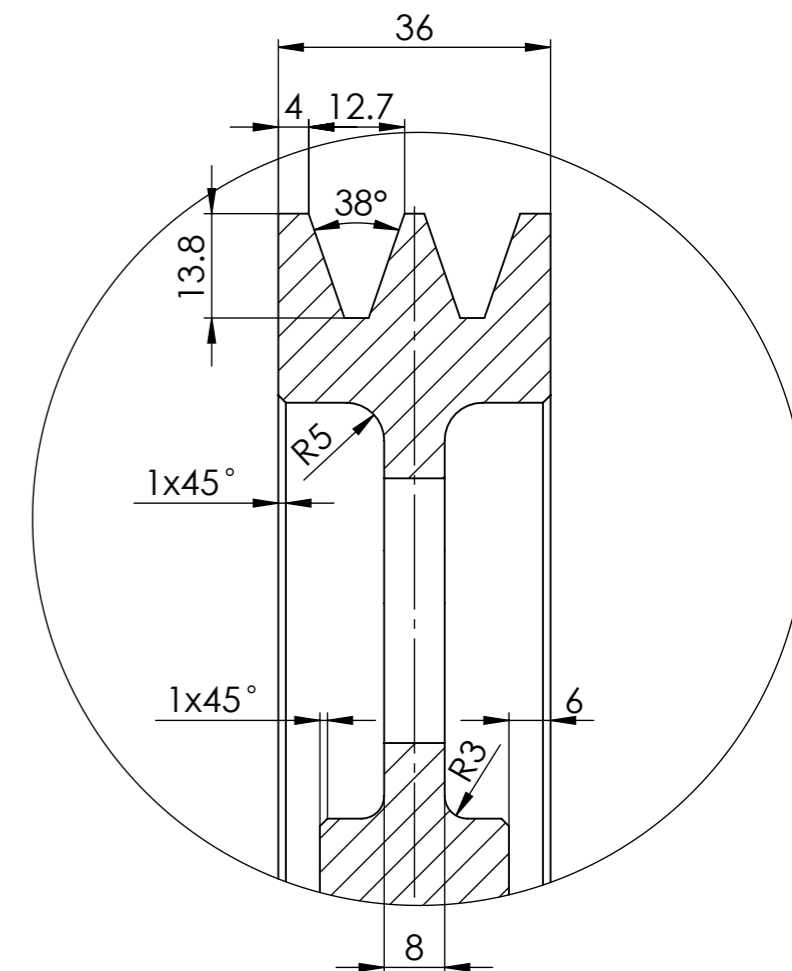
Detalj C Razmera 1 : 1
