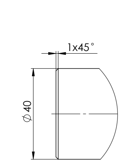
Detalj A Razmera 1 : 1
