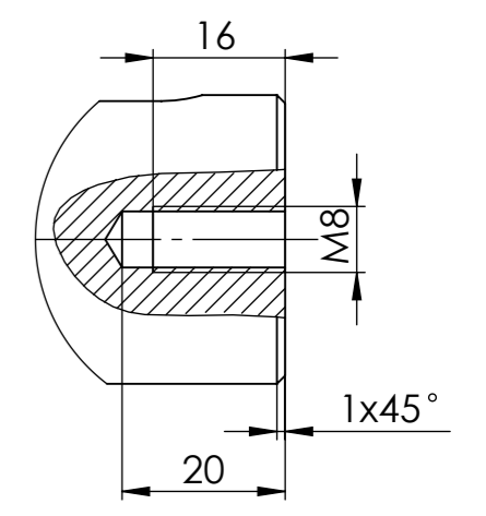
Detalj D Razmera 1 : 1
