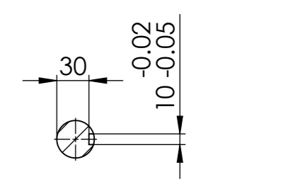
Detalj D Razmera 1 : 1
