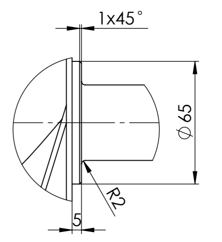
Detalj C Razmera 1 : 2
